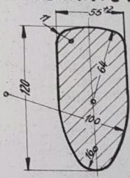
Schnitt C-D
